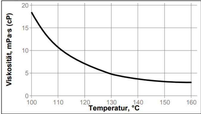
Temperatur/Viskositäts Profil:
